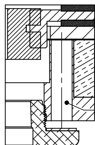
SEZIONE C-C
