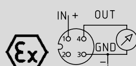
Stecker M12x1
