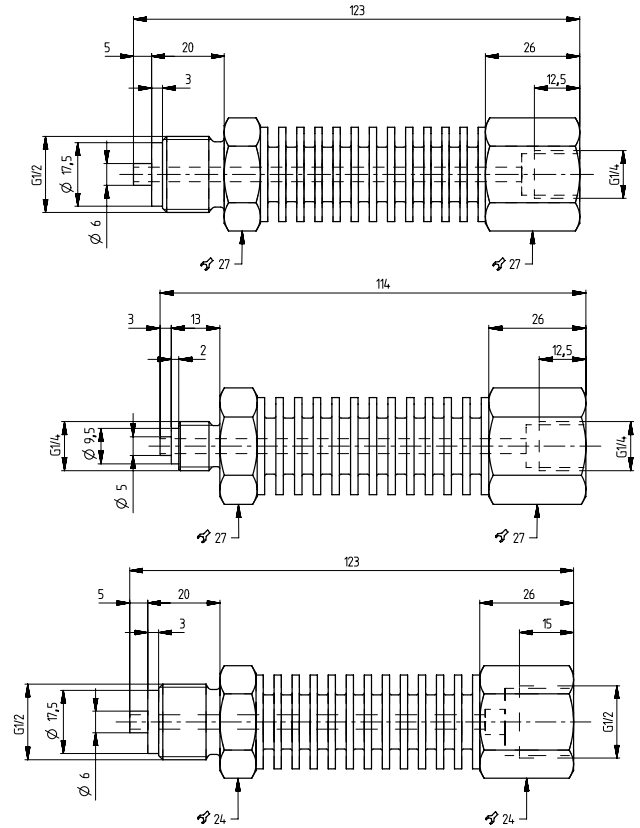
Kühlkörper
